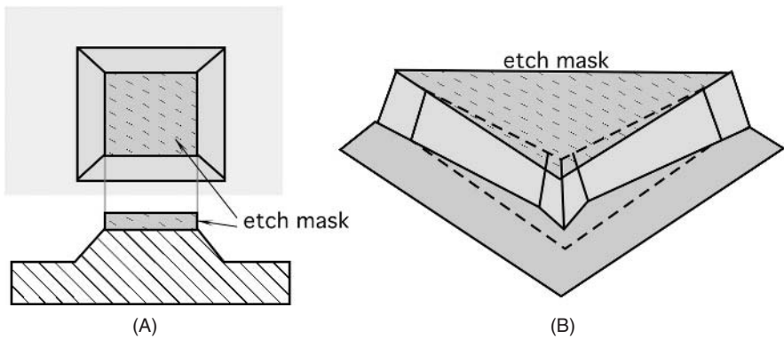
Fig. 18.11. Mesa structures.
